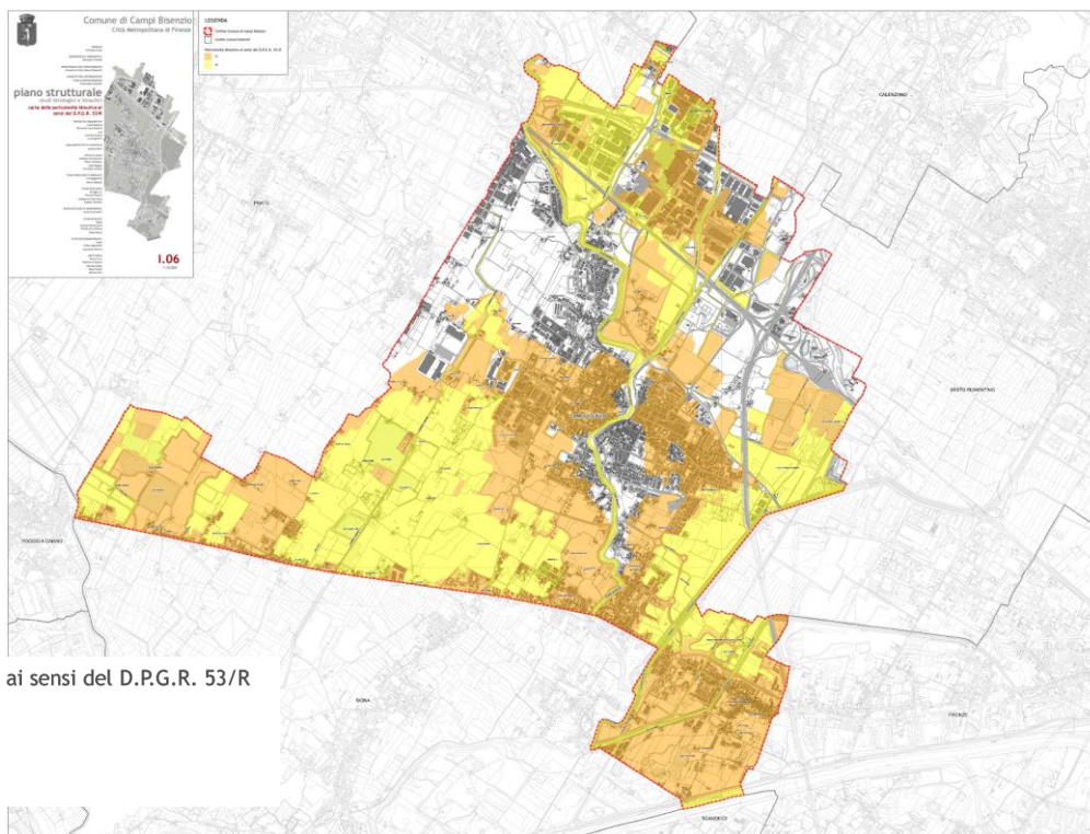
Pericolosità idraulica ai sensi del D.P.G.R. 53/R (PI6 del PS)
