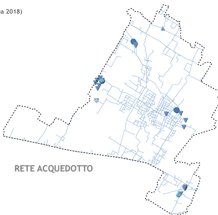
Rete acquedotto- Servizi a rete (QC.16)
