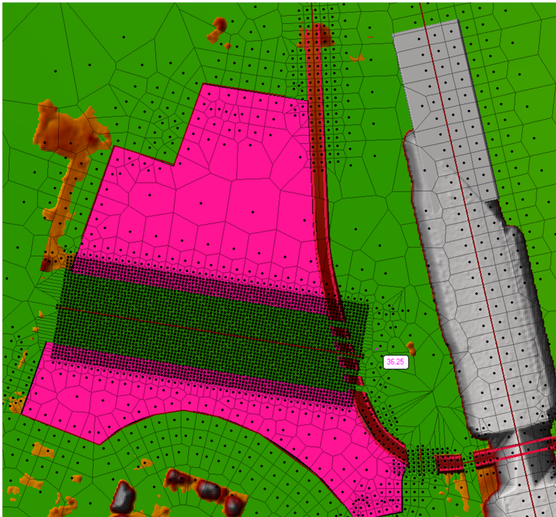
Figura 4 Risultati del modello idraulico in corrispondenza del Deposito S. Donnino
