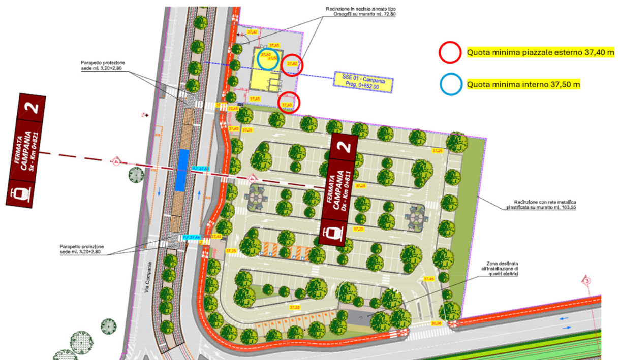
Figura 3 Parcheggio e SSE Elettrica Campania: sistemazione di progetto con evidenza delle quote della SSE
