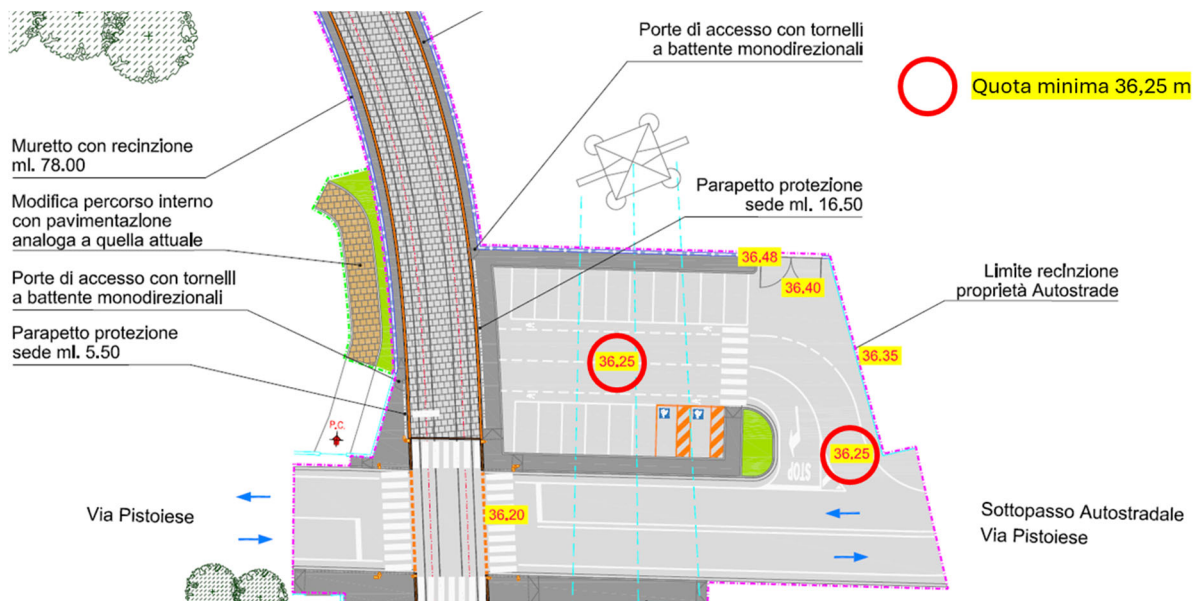
Figura 6 Parcheggio S. Donnino: sistemazione di progetto con evidenza delle quote del parcheggio
