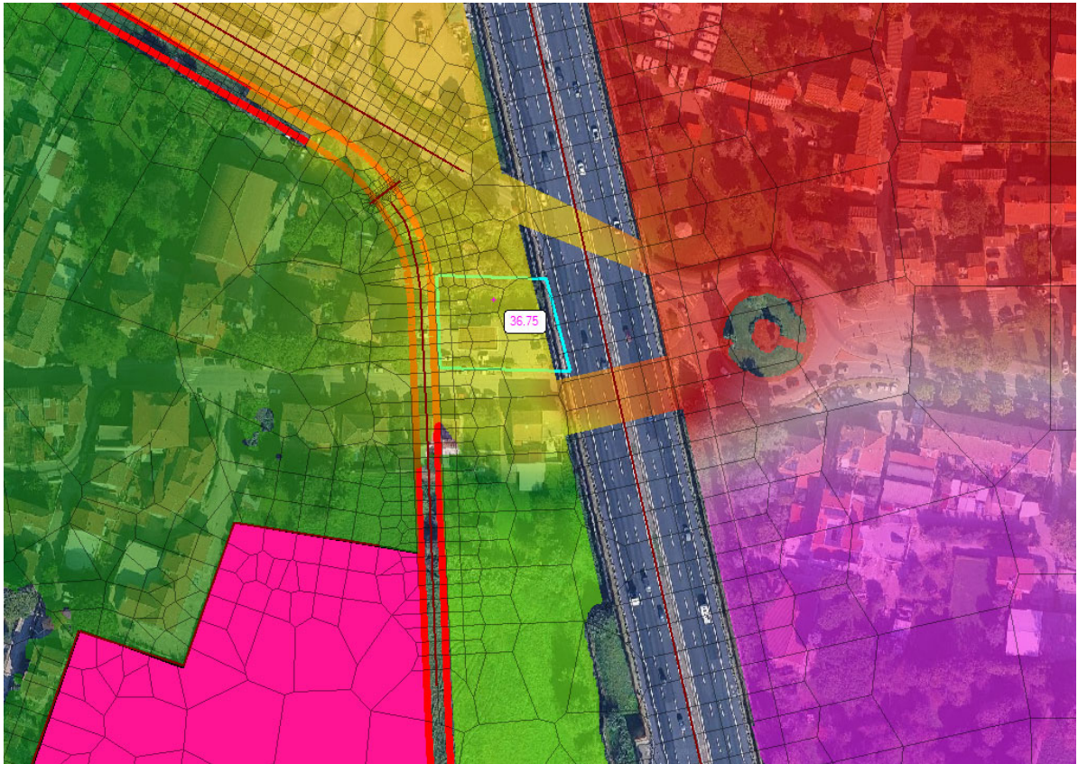
Figura 5 Risultati del modello idraulico in corrispondenza del Parcheggio S. Donnino
